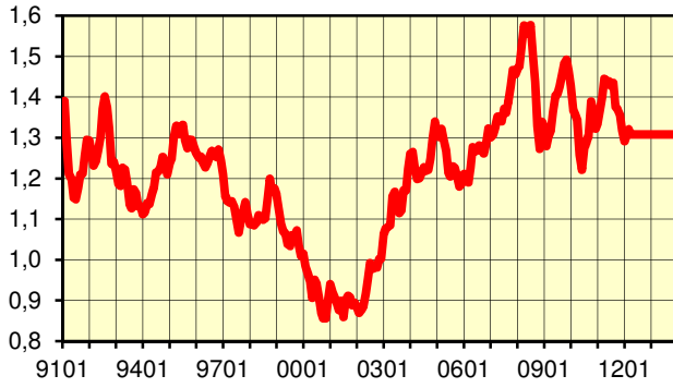
Växelkurs EUR/USD
